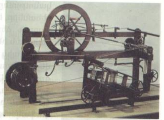
«Ջեննի» ձախարակ
