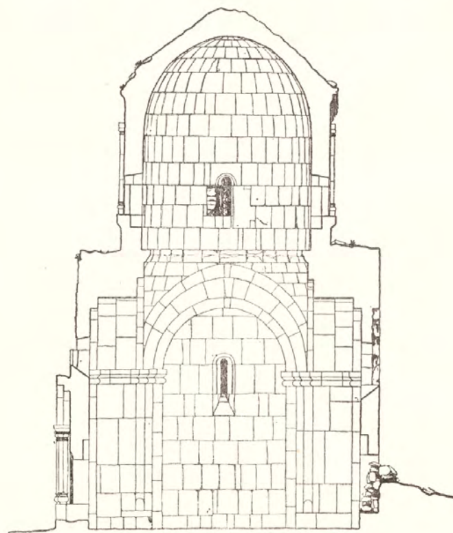
Գծ. 10. Եկեղեցու լալնական կտրվածքը։
