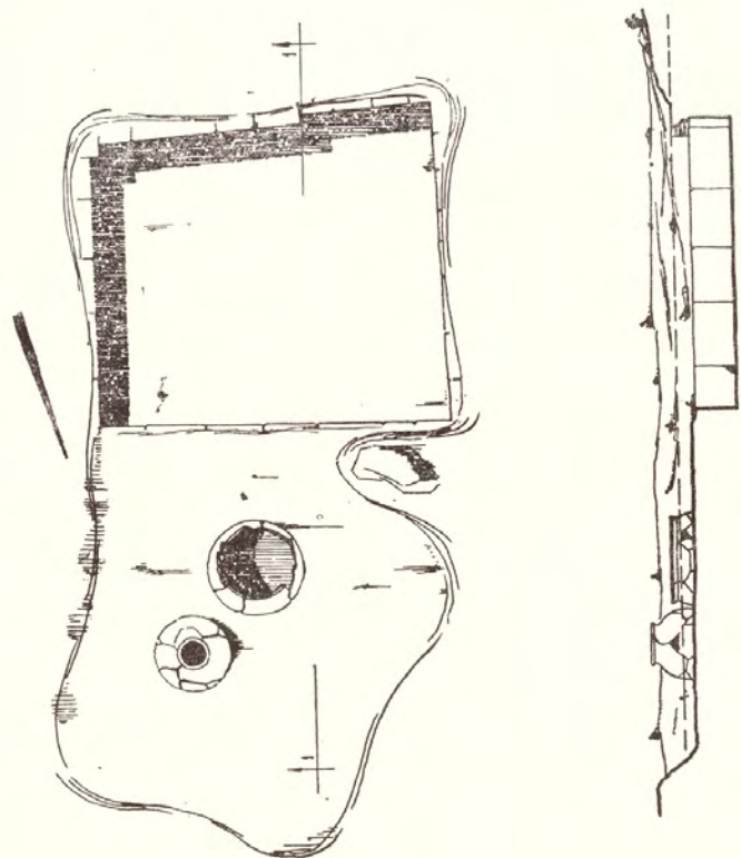
Գծ. 13. Ամրոցի հարավային մասում պեղված սենյակը:
