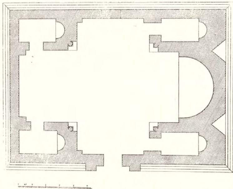
Գծ. 7. Եկեղեցու հատակագիծը:
