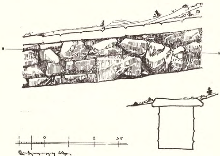
Պ. 6. Ամրոցի հարավային զաղտնուղին
