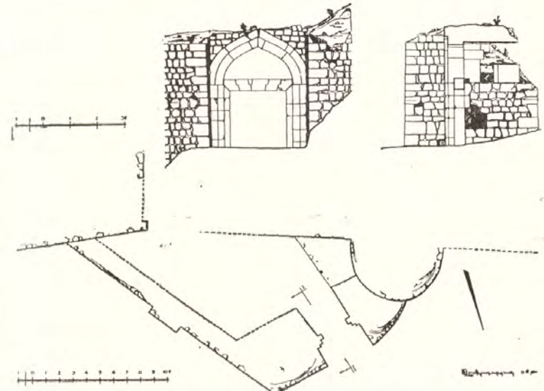
Գծ. 2. Արխաշանի դարբասը:
