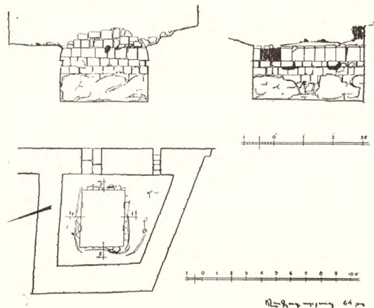
Գծ. 4. Միջնաբերդի ջրամբարը. հատակագիծ և կտրվածք:
