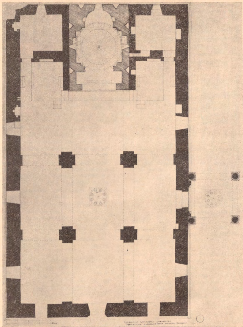
1. Կաթողիկէ եկեղեցու Հատակագիծը, ավագ խորանի տեղում Աստվածածին եկեղեցին Չափազրոյթուն՝ Տարագրոսի:
