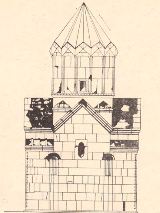
7. Նորաշայտ Աստվածածին եկեղեցու հր ճակատը: Զափագրություն՝ ՊԻ ուսանողների, զծագրեց՝ Զ. Գապուրյան:
