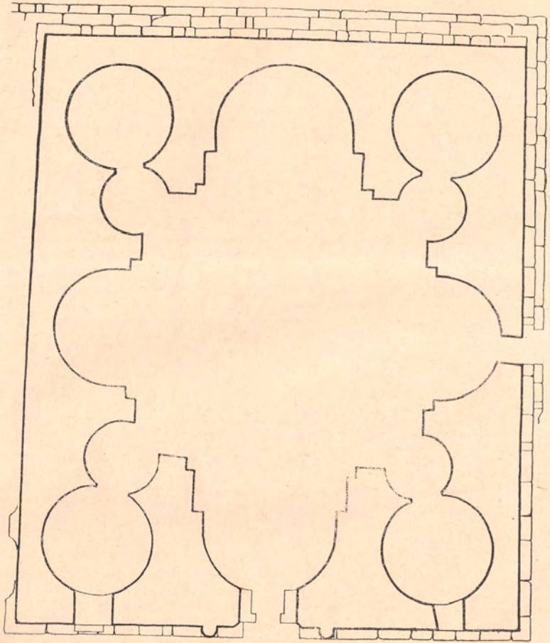
13. Ավանի տաճարի հասակաձևը Չափագրություն՝ Շ. Ազատյանի:
