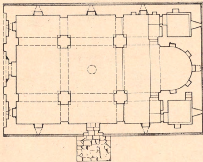
28. Քանաքեռի՝ ս. Աստվածածին եկեղեցու հատակածեր և կորվածքը: Չափագրության՝ Կուչյան Ղաֆադարյանի:
