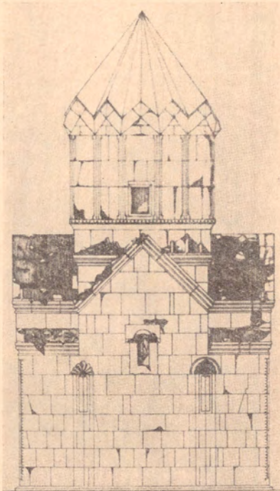
4. Նորահայտ Աստվածածին եկեղեցու հա հատար: Չափազորություն՝ 9/16 ուսանդների, զծաղրեց՝ 2. Գապարչյան:
