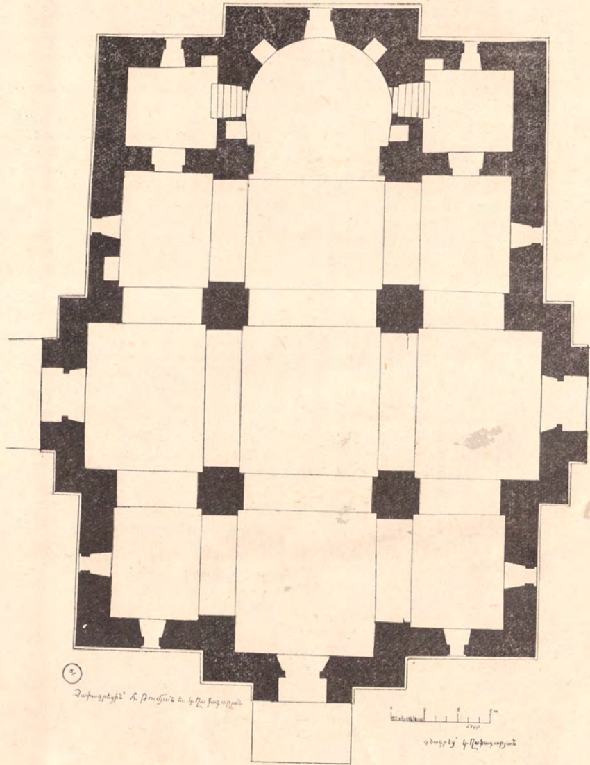
29. Նորի Սիմեոն Սերունի էկզեկցու հատակակերտ Չափադրույթուն՝ Կարա Ղաֆաղաբյանի և Հարություն Քումյանի:
