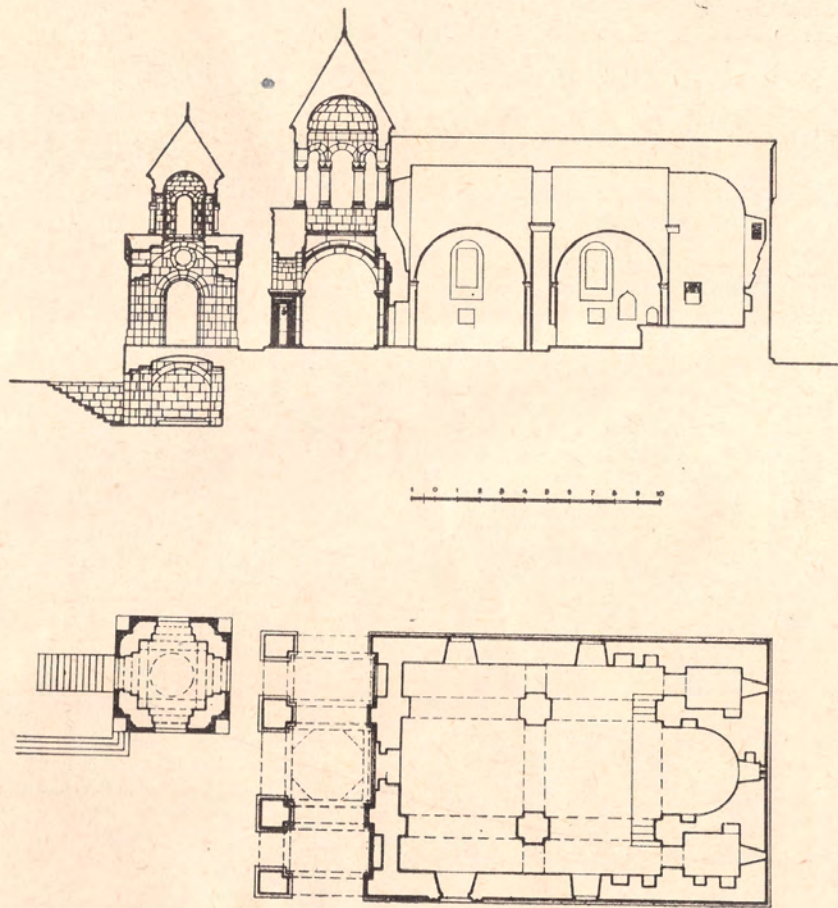
8. Զորավոր եկեղեցու հատակածեր և երկարության կտրվածքը: Չափազրոյւթիւն՝ Կորյուն Գափաղաւանի:
