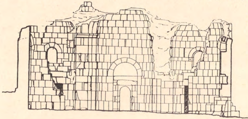
19. Ավանի տաճարի զեպի ամ կորվածքը: Չափազորություն՝ 5. Ազատյանի:
