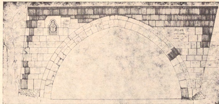
10. Նորբի կամուրջի հր ճակատը 1965 թ. վերանորոգումից հետո (ներկայացվում է վերանորոգման նախագիծը): Չափազրույթյուն՝ Շ. Ազատյանի և Յու. Քամանյանի:
