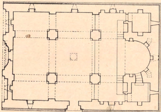
27. Քանաքեռի ս. Հակոբ եկեղեցու հատակածեր և կորվածքը: Չափագրության՝ Կուչյան Ղաֆադարյանի:
