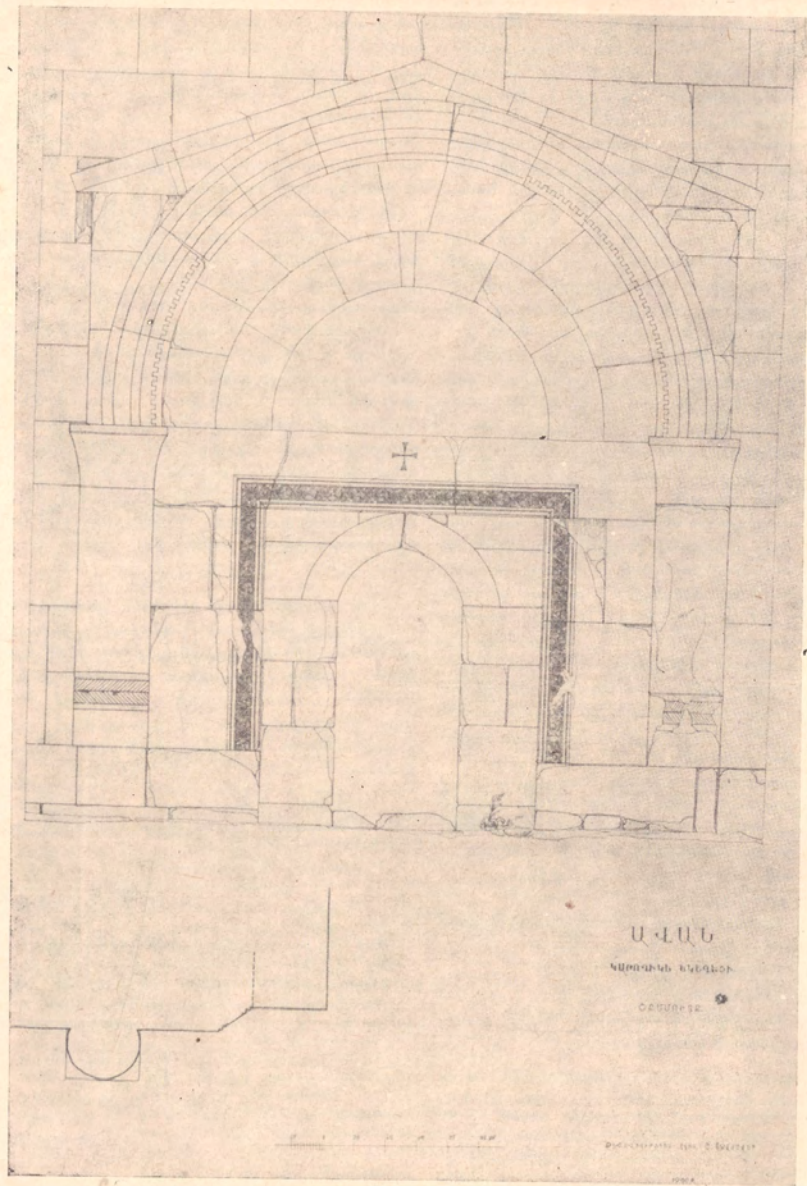
22. Ավանի տաճարի ամ մուտքի ճակատը: Չափազրույթյուն՝ Շ. Ազատյանի:
