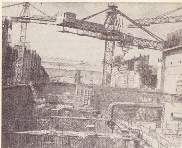
Строительство Евфратской плотины
