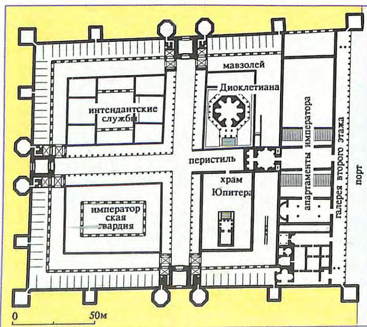
3 ПЛАН ДВОРЦА ДИОКЛЕТИАНА
