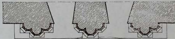
ГОШАВАНК ЦЕРКОВЬ СВ. ПРОСВЕТИТЕЛЯ ВОСТОЧНОЕ ОКНО
