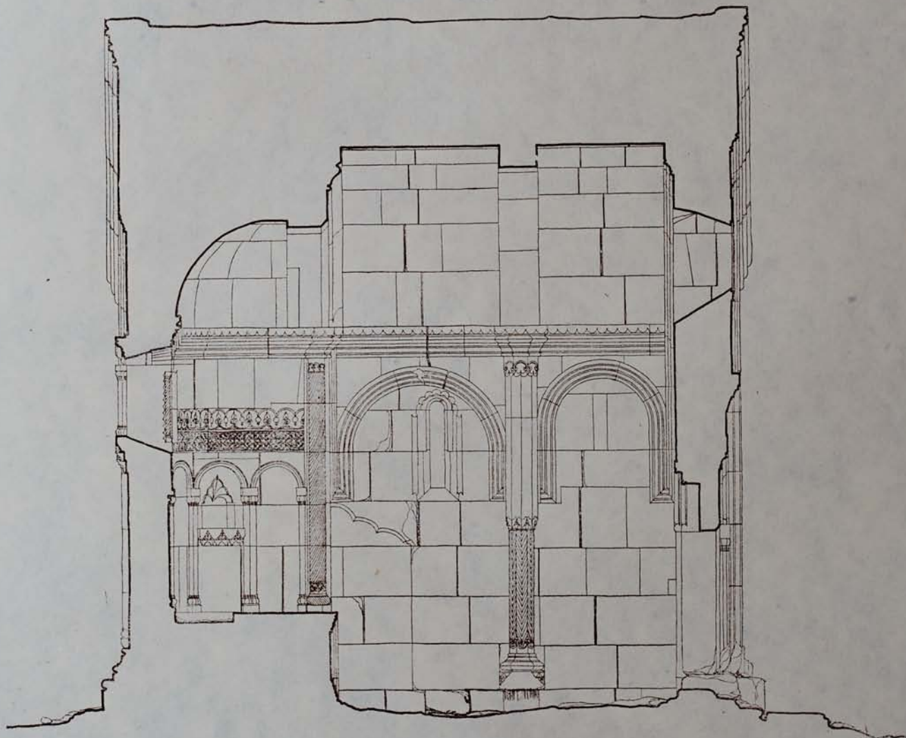
ԳՈՏԱՎԱՆԻ Ս. ԼՈՒՍԱՎՈՐԻՉ ԵԿԵՂԵՑԻ ԸՆԴԵՐԿԱՑՆԱԳԱՆ ԿՏՐՎԱՆԻՔ
