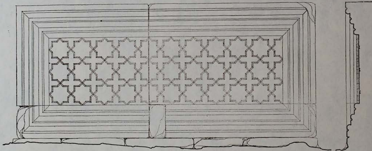
ГОШАВАНК ЦЕРКОВЬ СВ. ПРОСВЕТИТЕЛЯ ДЕТАЛИ АПСИДЫ
