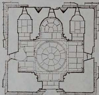
ЦЕРКОВЬ СВ. ГЕОРГИЯ ПЛАН, ПЛАФОН И КРОВЛЯ
