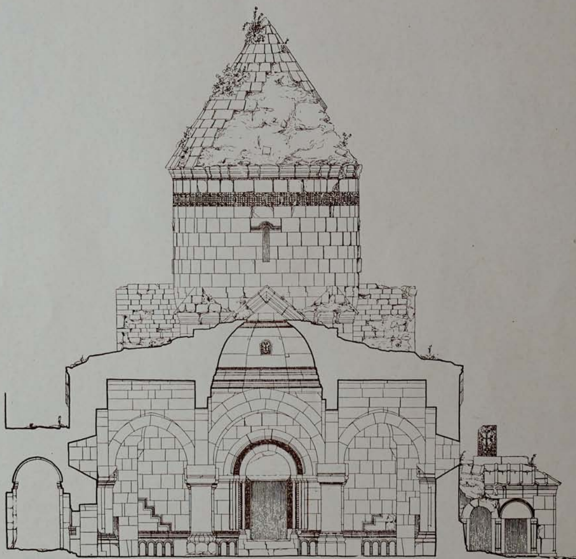
ԳՈՏԱՎԱՆԿ Ս. ԱՍՏՎԱԾԱԾԻՆԻ ԵՎ ԲՆԻՎՈՒՄԻ ԸՆԴՀԱՆՈՒՄԻ ԱՏՐՎԱԾԻ
