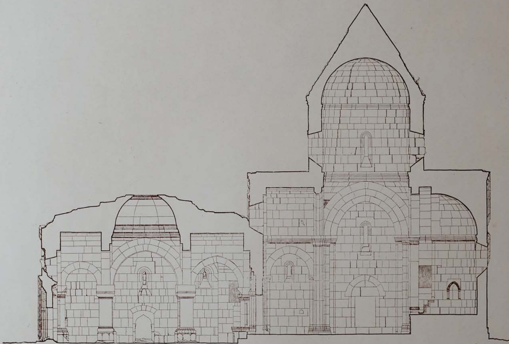
ГОШАВАНК ЦЕРКОВЬ СВ. БОГОРОДИЦЫ И ПРИТВОР ПРОДОЛЬНЫЙ РАЗРЕЗ
