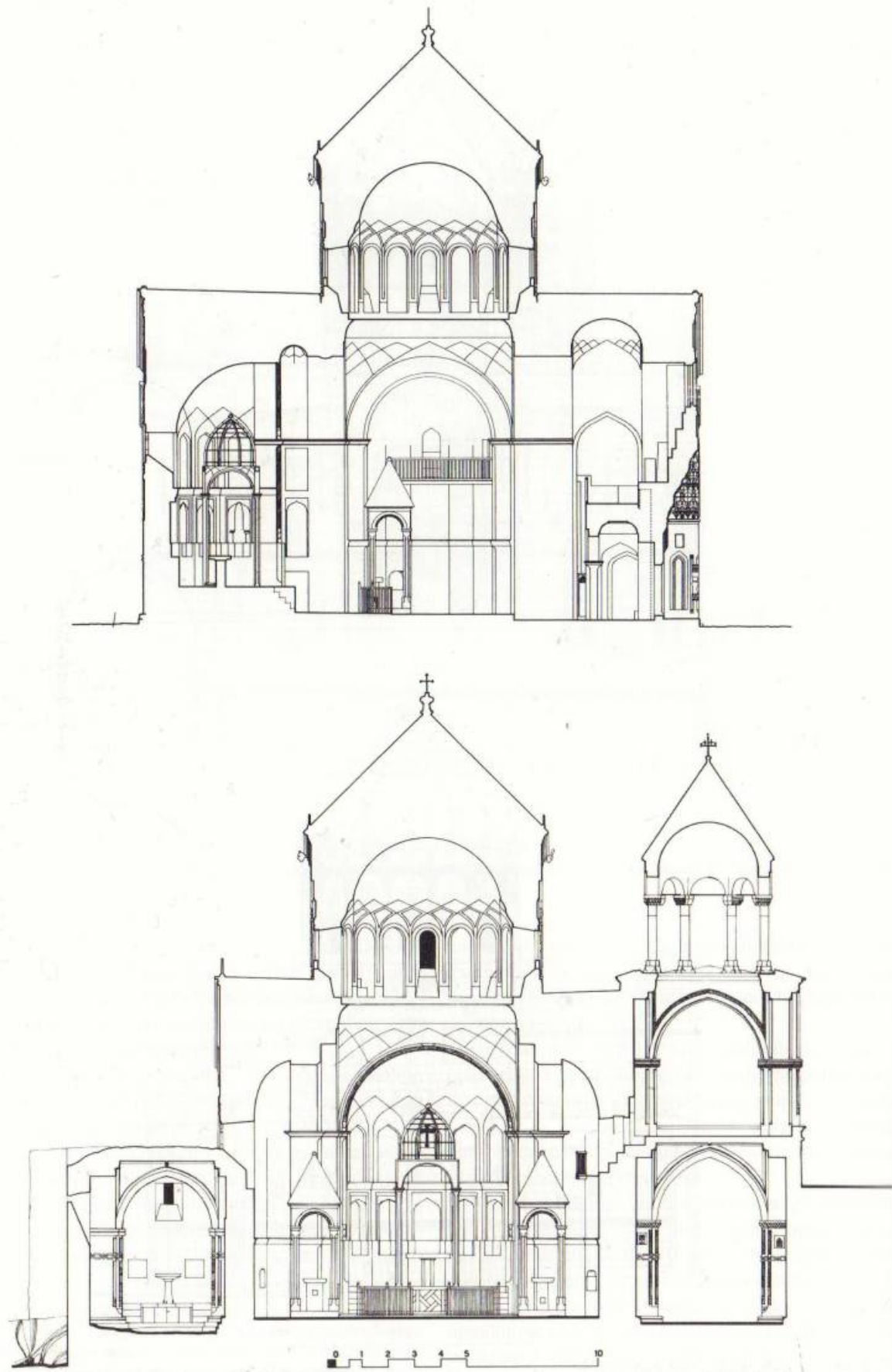
Մաղարղավանքի Սր. Ստեփանոս եկեղեցու կտրվածքը դեպի հարավ և արևելք (չափ.՝ ճարտ. դր. Գարբնուտ Գոֆրիխտերի)
