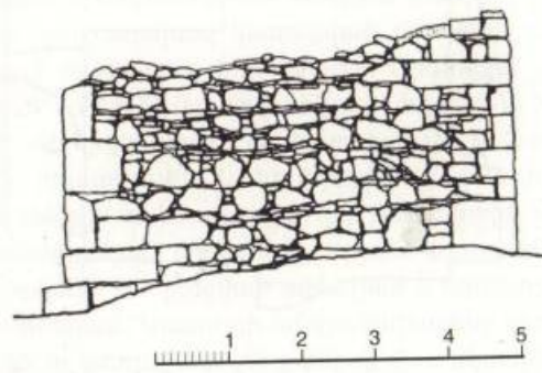
Սք. Աստվածածին կամ Նահատակության տեղի փոքր մատուռի հատակագիծն ու հարավային ճակատը (չափ.՝ ճարտ. դր. Արմեն Գալստյանի)
