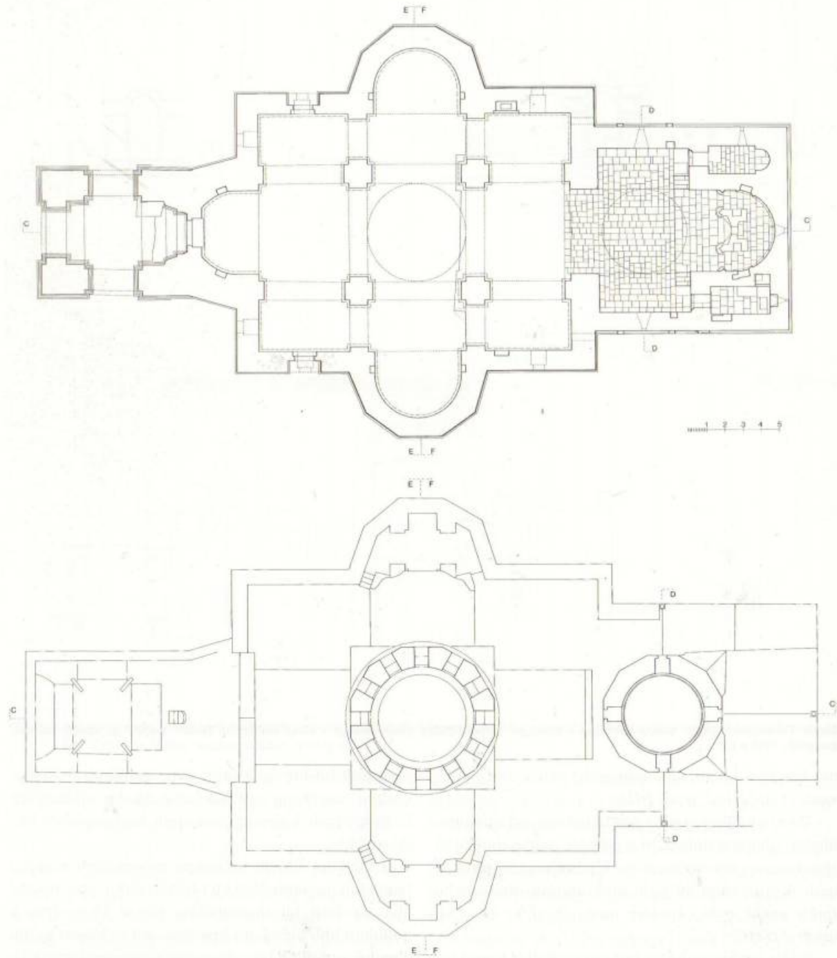
Թաղեոս առաքյալի վանք. գավիթ-եկեղեցու և եկեղեցու կտրվածքները դեպի արևելք և դեպի արևմուտք (չափ.՝ ճարտ. դր. Արմեն Գախնազարյանի, 1988 թ.)
