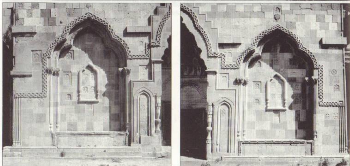
Մաղարդավանքի Աբ. Ստեփանոս եկեղեցու արևմտյան ճակատից բացված մուտքը և հատվածներ նույն ճակատից (լուս.՝ ճարտ. դր. Արմեն Գալստյան)
