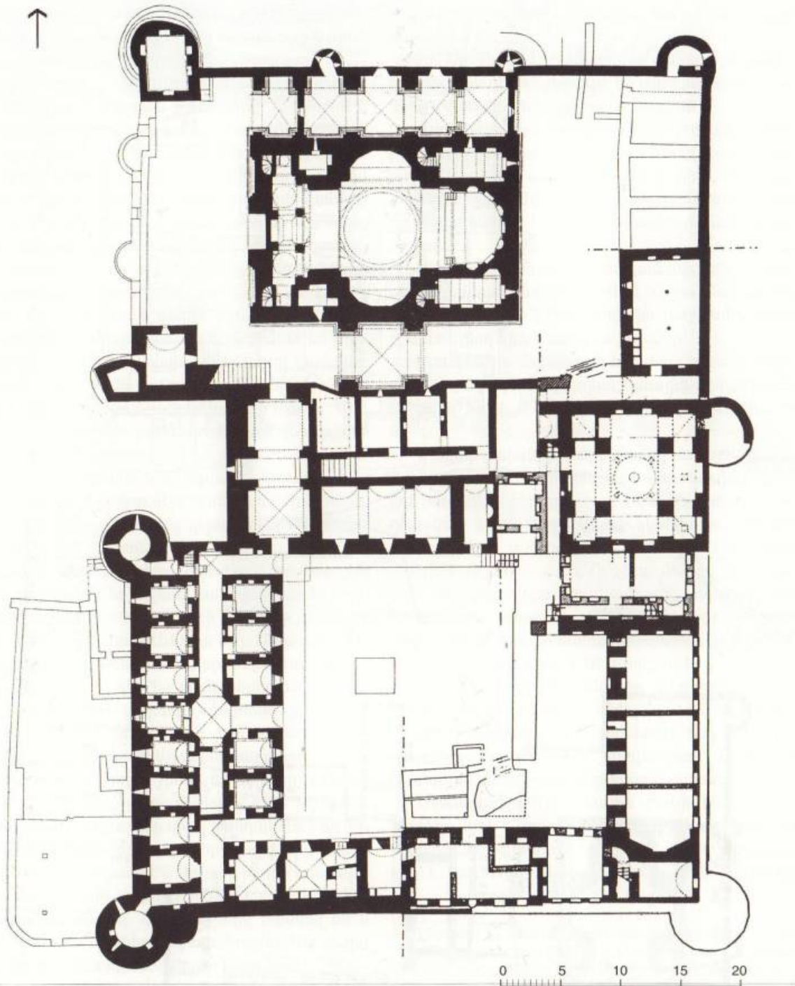
Մաղարդա Սր. Ստեփանոս ճախավկայի վանքի գլխավոր հատակագիծը (չափ.՝ ճարտ. դր. Գարրծուտ Գոֆրիխտերի)
