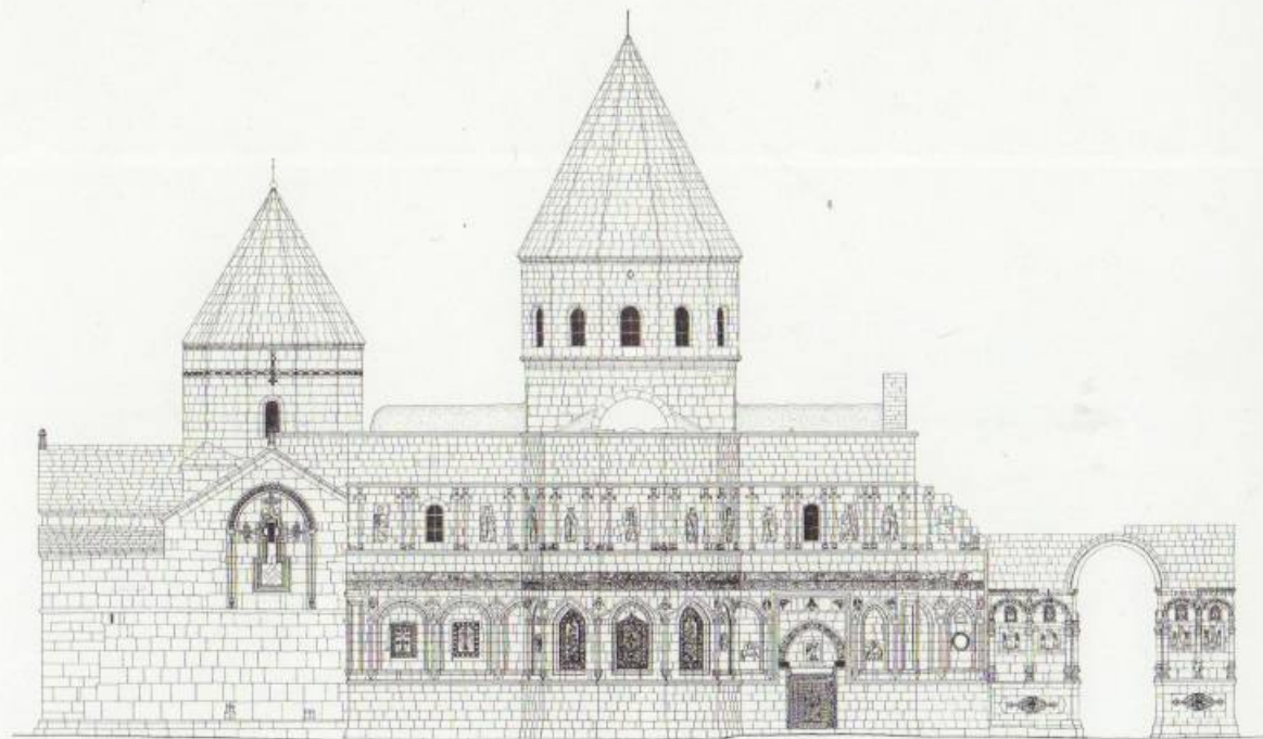
Թաղեոս առաքյալի վանք. եկեղեցու, գավիթ-եկեղեցու և զանգակատան հարավային և հյուսիսային ճակատները (չափ.՝ ճարտ. դր. Արմեն Գախնազարյանի, 1968 թ.)
