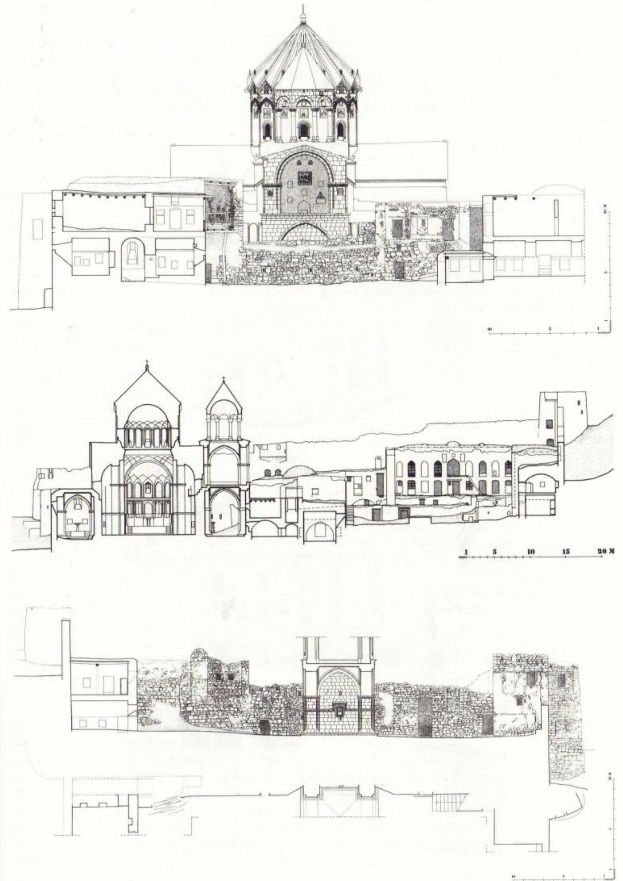
Մաղարղա Սր. Ստեփանոս մախավկայի վանքի լայնակի կտրվածքները դեպի հյուսիս, արևելք և հարավ (չափ.՝ ճարտ. դր. Գարբնուտ Գոֆրիխտերի)
