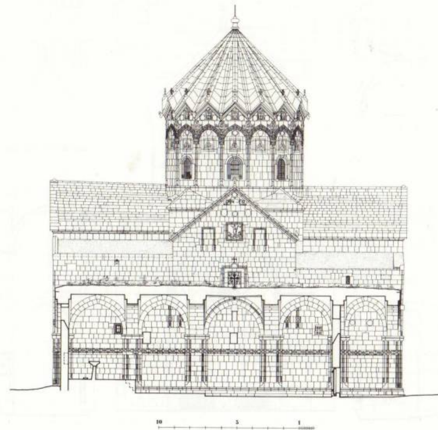
Մաղարդավանքի Աբ. Ստեփանոս եկեղեցու հարավային և հյուսիսային ճակատները (չափ.՝ ճարտ. դր. Գարթմուտ Գոֆրիխտերի)
