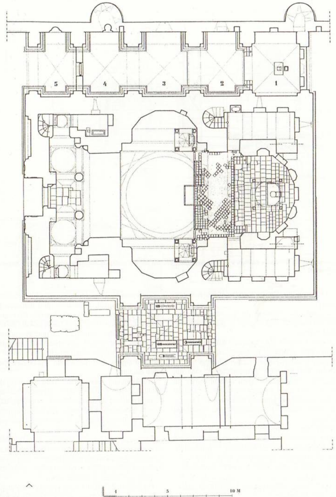
Մաղարդա Սր. Ստեփանոս ճախավկայի վանքի զույգ եկեղեցիների և հարակից կառույցների հատակագիծը (չափ.՝ ճարտ. դր. Գարրծուտ Գոֆրիխտերի)
