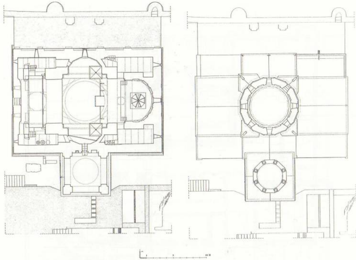
Մաղարդավանքի Սր. Ստեփանոս եկեղեցու և հարակից կառույցների երկրորդ հարկի և տանիքի հատակագծերը (չափ.՝ ճարտ. դր. Գարրոնուտ Գոֆրիխտերի)
