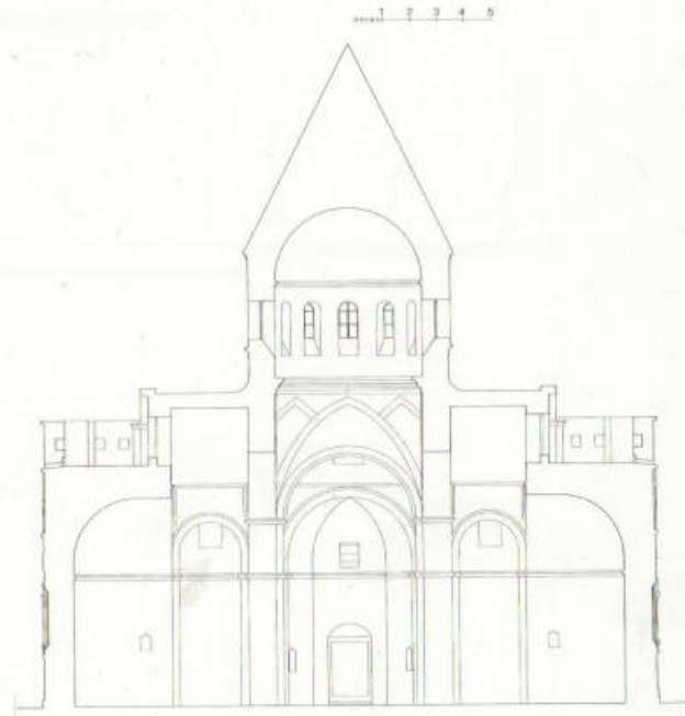
Թաղեոս առաքյալի վանք. գավիթ-եկեղեցու և եկեղեցու կտրվածքները դեպի արևելք և դեպի արևմուտք (չափ.՝ ճարտ. դր. Արմեն Չախնազարյանի, 1968 թ.)
