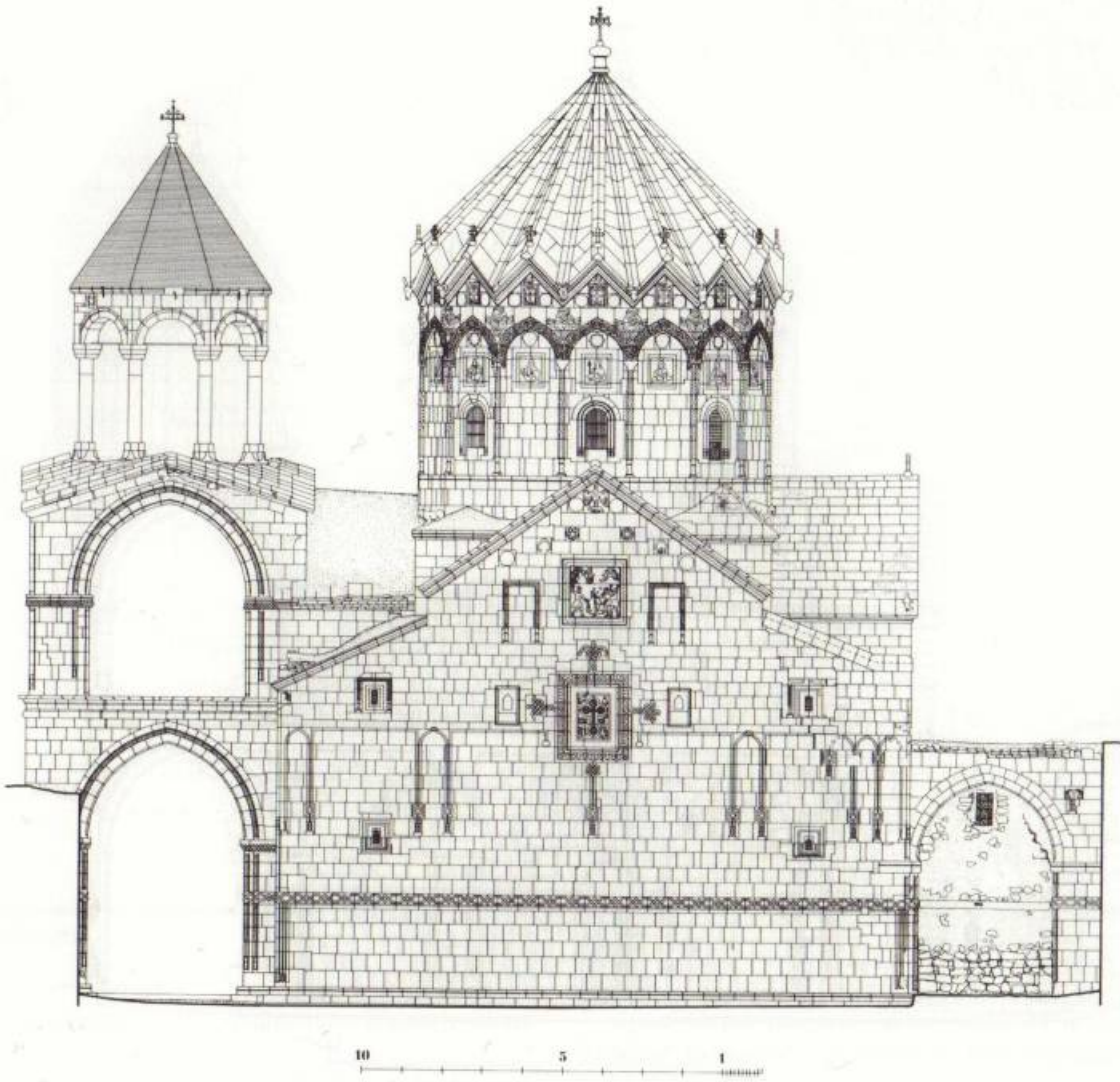
Մաղարդա Աբ. Ստեփանոս նախավկայի վանքի եկեղեցիների և զանգակատան արևելյան ճակատը (չափ.՝ ճարտ. դր. Գարթմուտ Գոֆրիխտերի)
