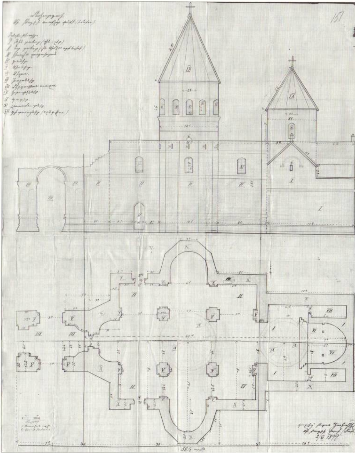
Թաղեռն առաքյալի վանք (չափ.՝ ճարտ. Թարոս Ղազարյանի, 1899 թ.)
