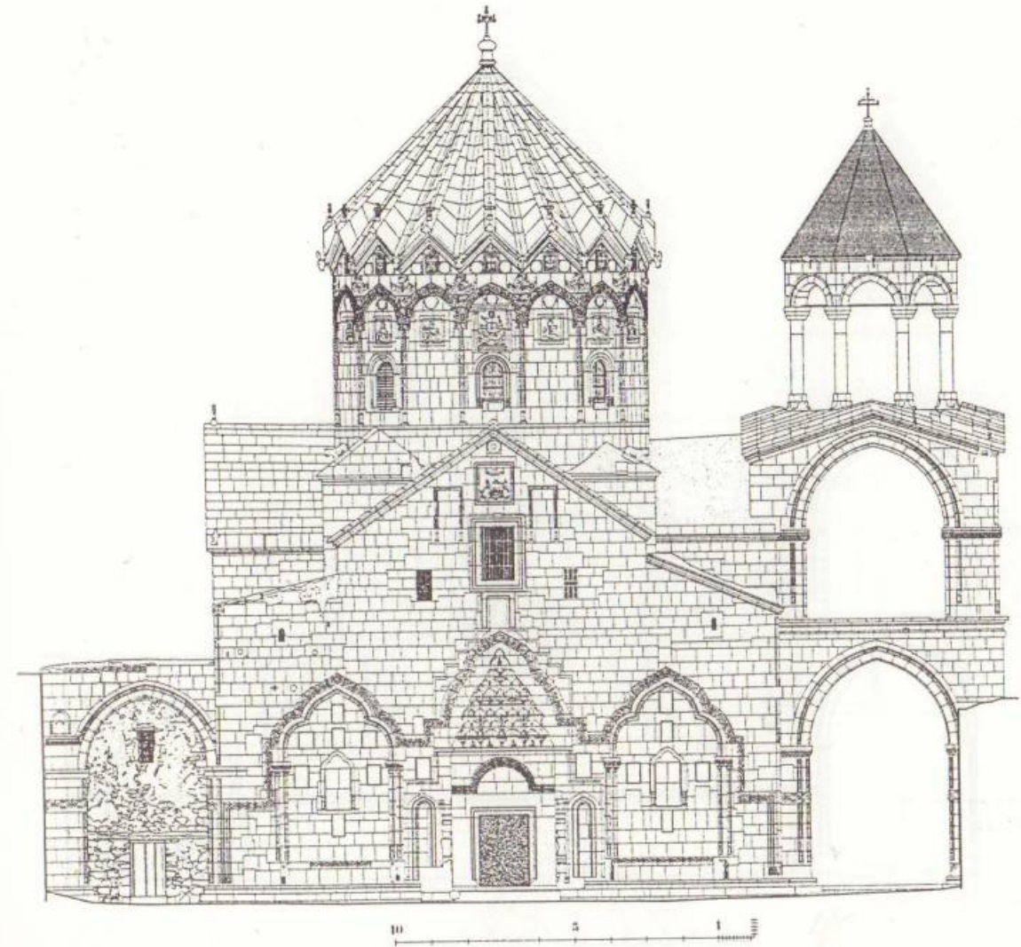
Մաղարդա Սր. Ստեփանոս մայրավայրի վանքի եկեղեցիների և զանգակատան արևմտյան ճակատը (չափ.՝ ճարտ. դր. Գարրոնուտ Գոֆրիխտերի)
