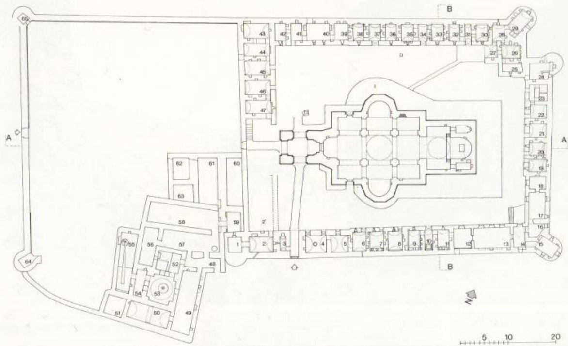
Թաղեոս առաքյալի վանք. համալիրի գլխավոր հատակագիծը (չափ.՝ ճարտ. դր. Արմեն Գախնազարյանի, 1968 թ.)
