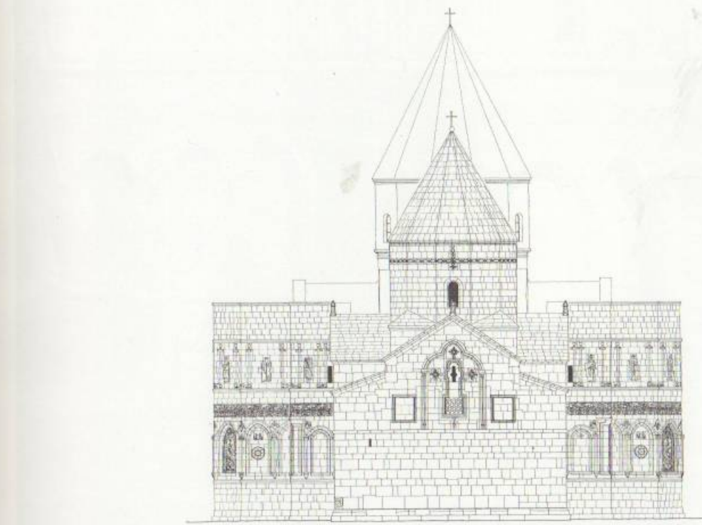
Թաղեոս առաքյալի վանք. կենտրոնական կառույցների արևմտյան և արևելյան ճակատները (չափ.՝ ճարտ. դր. Արմեն Գախնազարյանի, 1968 թ.)
