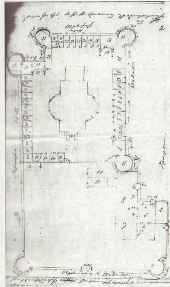
Խաչիկ ծ. վարդապետ Դադյանի կազմած Թադեոս առաքյալի վանքի հատակագիծը (1894 թ.)
