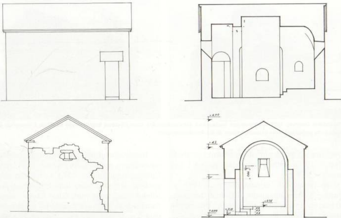
Սր. Սանդուխտ մատուռի հարավային և արևմտյան ճակատները և կտրվածքները դեպի հյուսիս և արևելք (չափ.՝ ճարտ. դր. Արմեն Գալստյանի)
