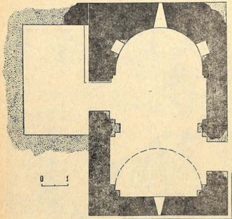
Рис. 9. План церкви св. Богородицы с. Кунгют.
