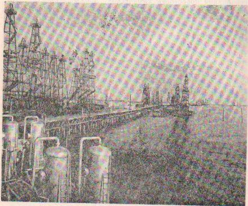
Участок 4-го промысла НПУ «Гюргяннефть».
