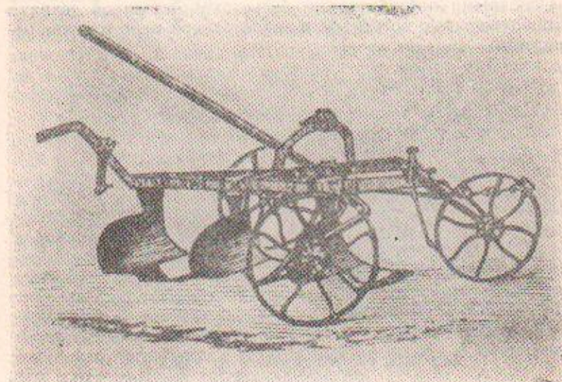
Трехкорпусный плуг Гена.
