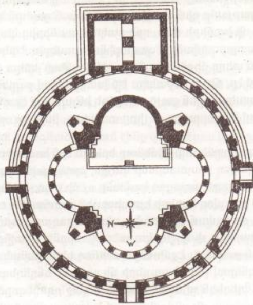
Զվարթնոց եկեղեցու հատակագիծը
